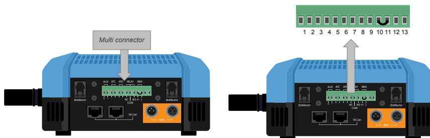
Placering av multi-kontaktdon
