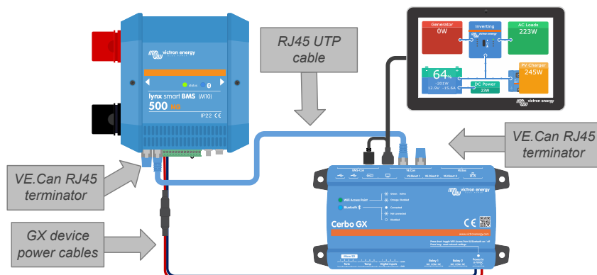
Kopplingsexempel Lynx Smart BMS NG och en Cerbo GX med GX Touch
