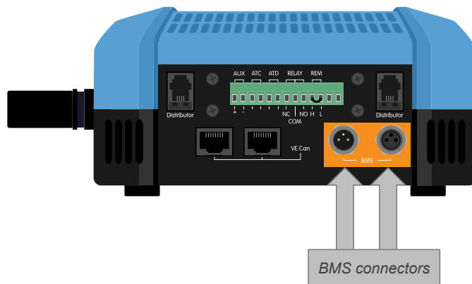
Placering av BMS-kabelkontaktdon
